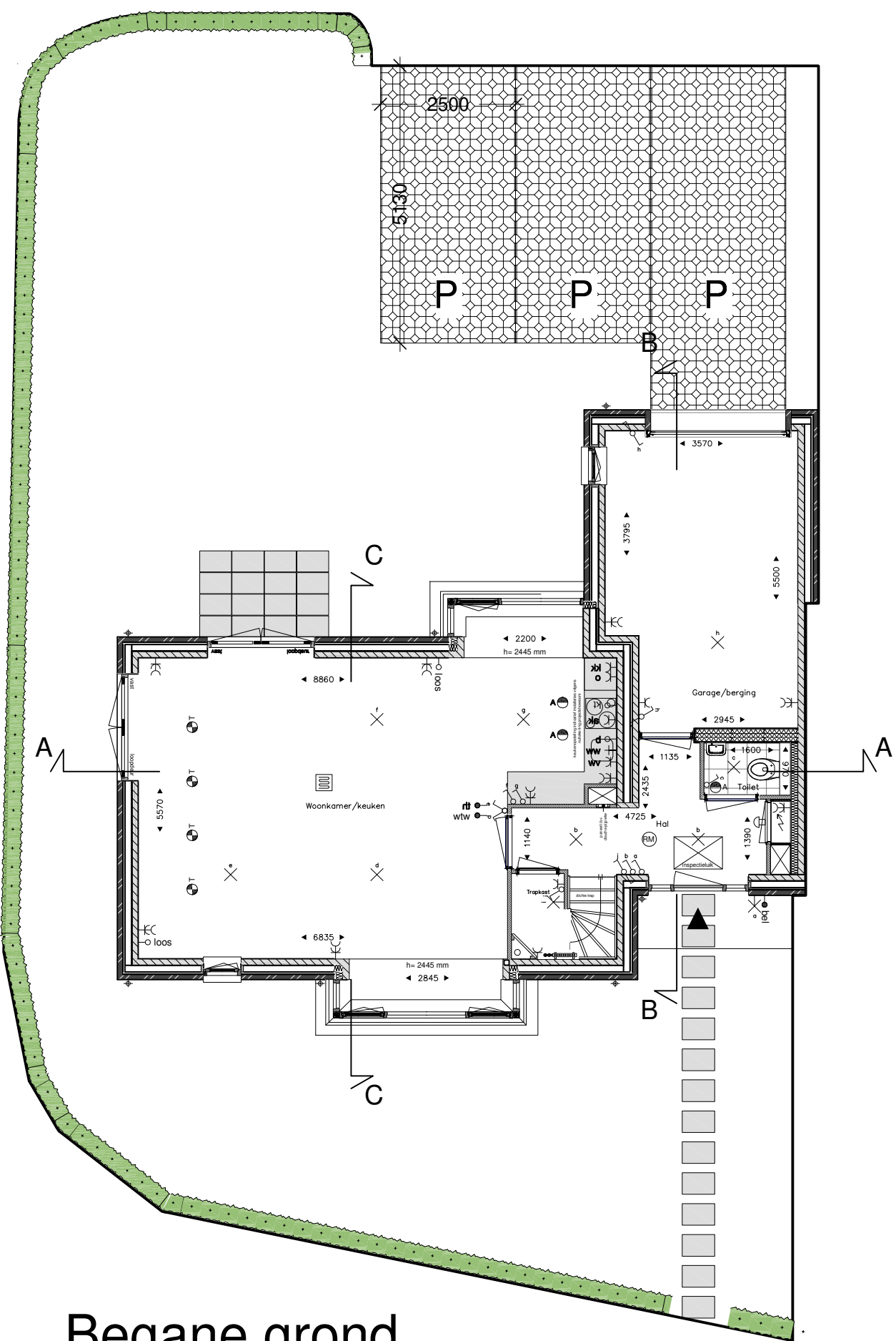
Begane grond
