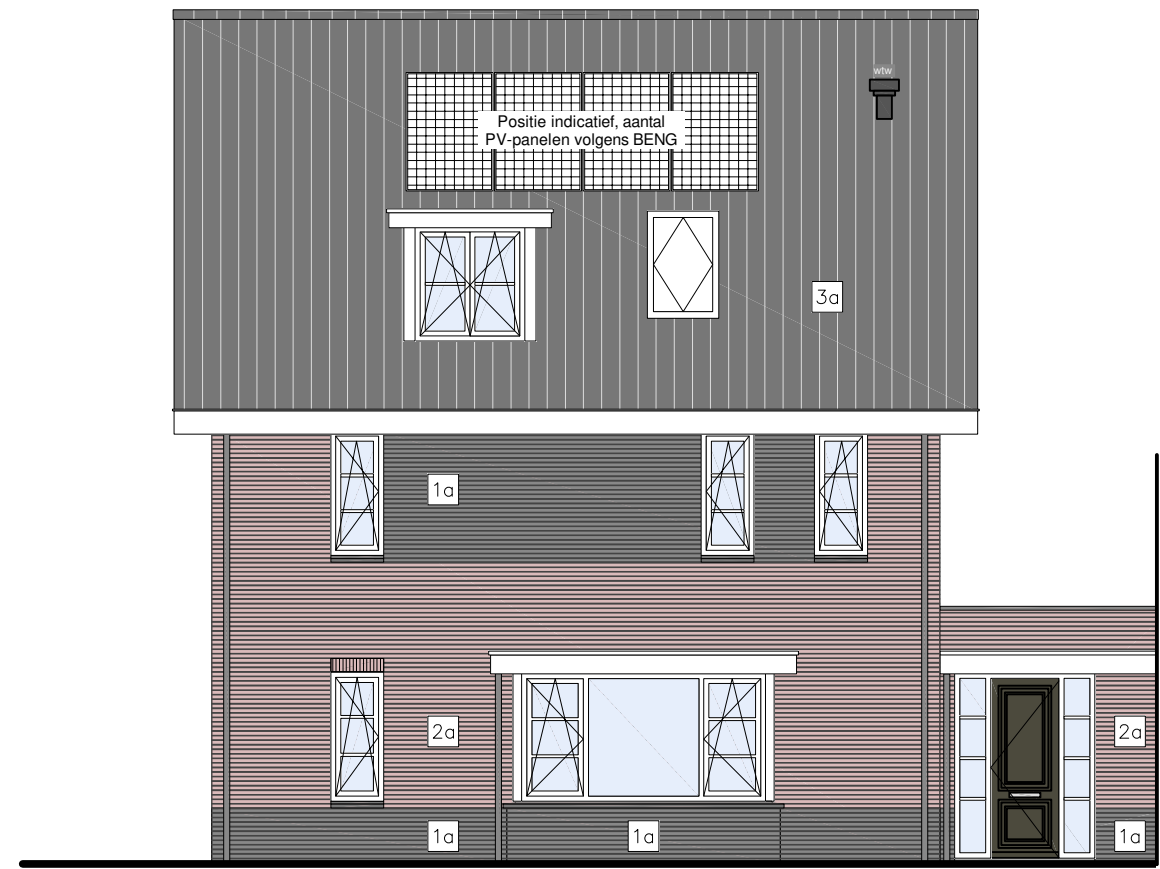
Zuidgevel
