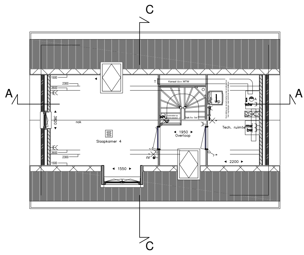
2e verdieping
