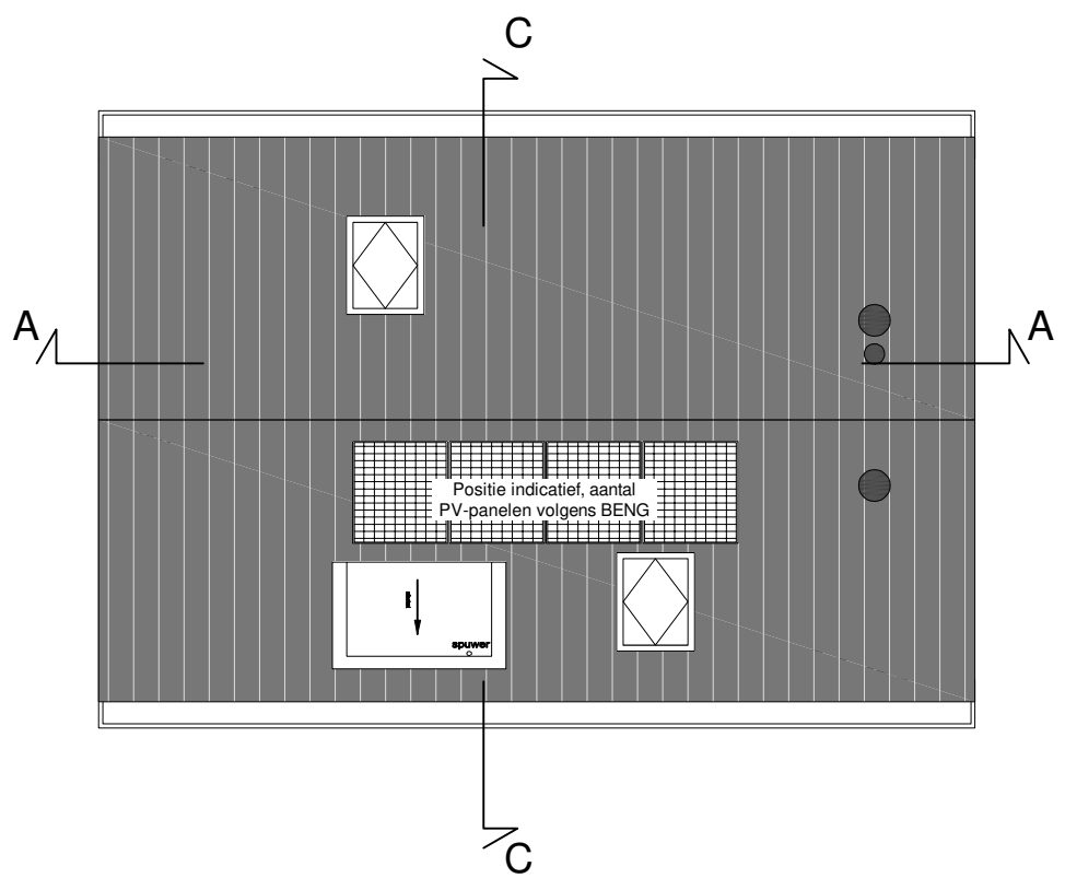
Dakaanzicht
