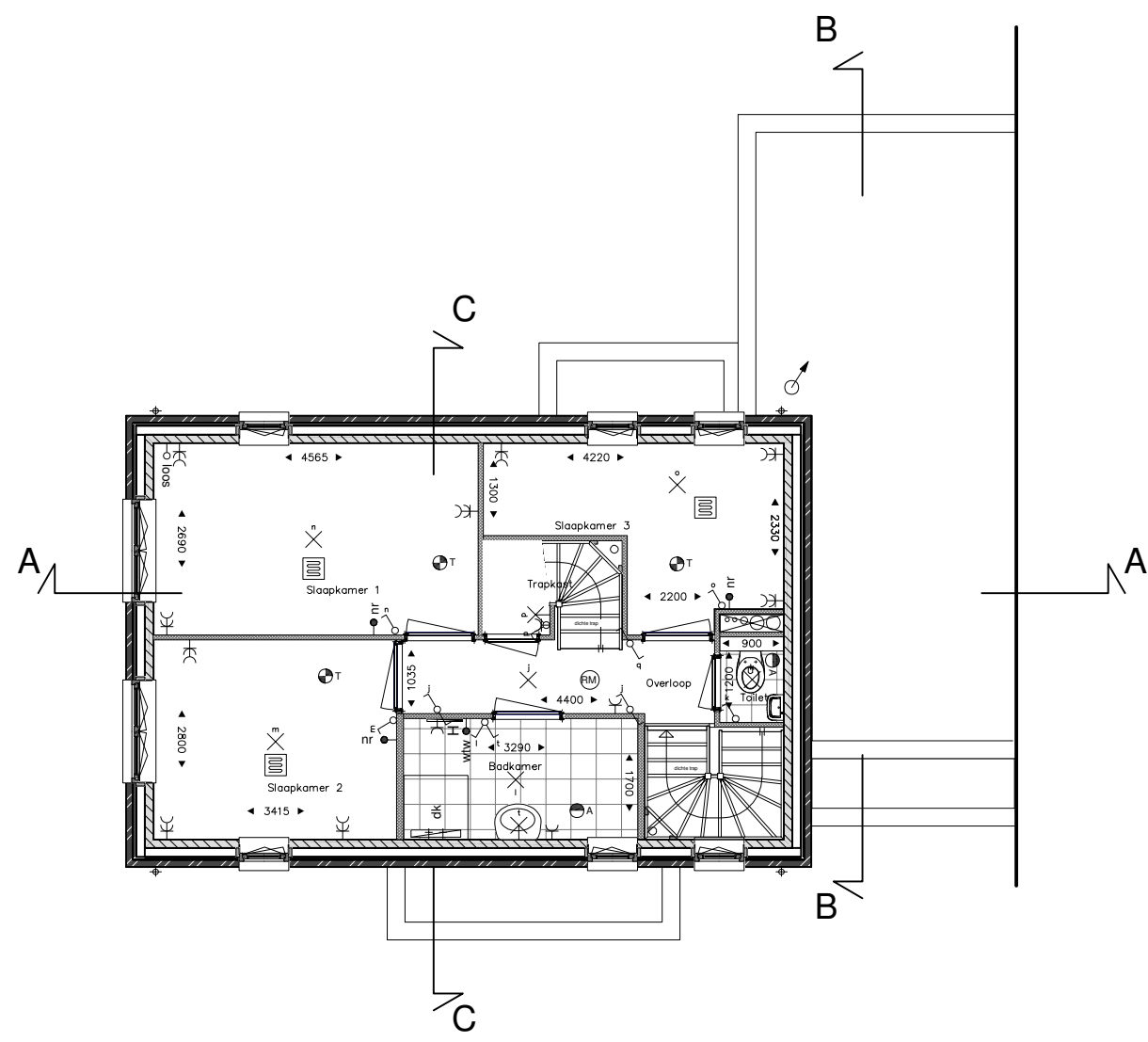
1e verdieping
