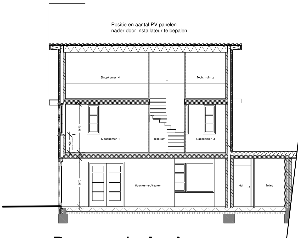
Doorsnede A - A
