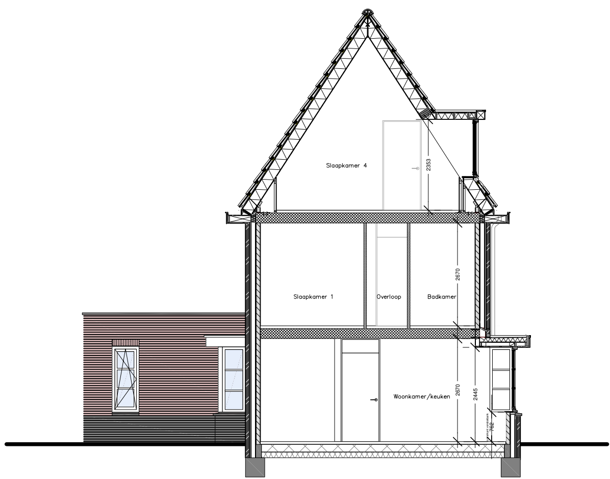
Doorsnede C - C
